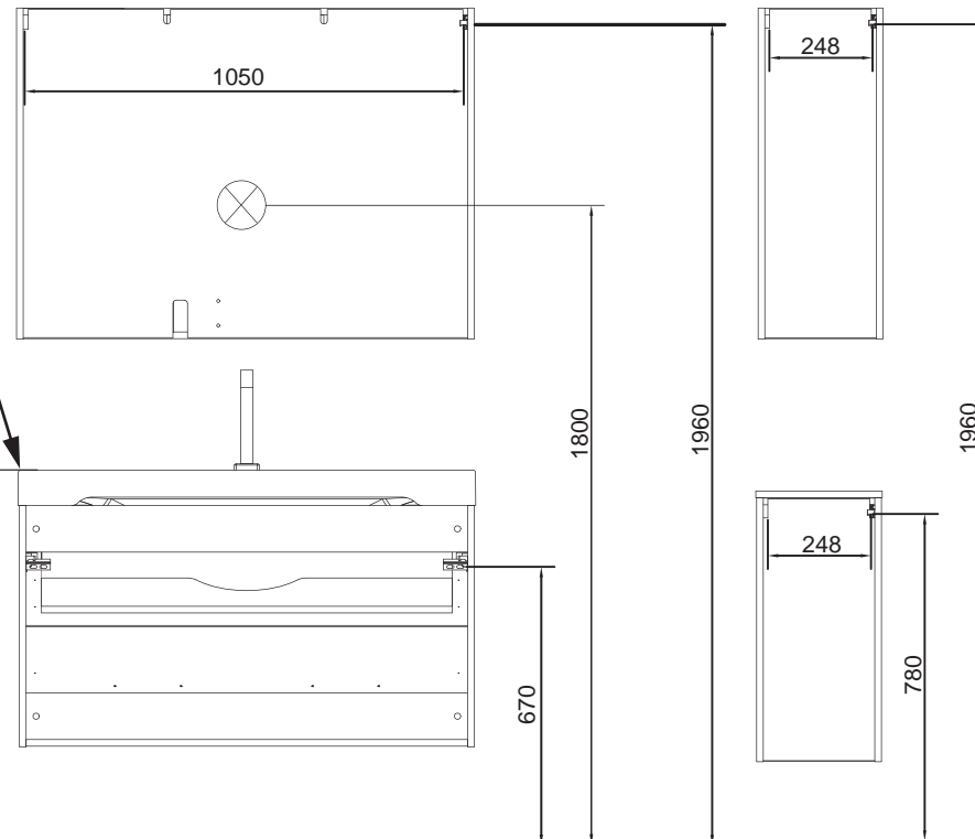
Ansicht Rückseite
